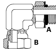
UNOM x BSPPFS 90° Elbow
