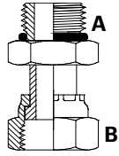
UNOM x ORFSFS Adaptor
