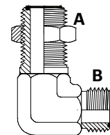
ORFSBH x ORFSM 90° Elbow
